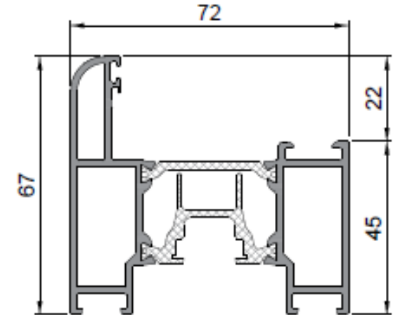
Door sash/vent
